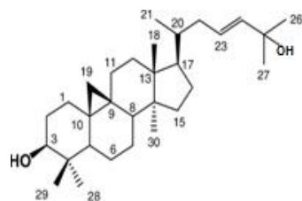
ترکیب ۲: سیکلوآرتان-۲۳-ان-۱-۳- \beta - \text{OH}
