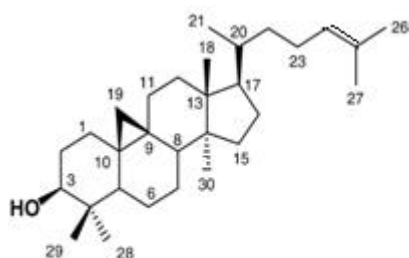
ترکیب ۴: سیکلوآرتان-۲۴-ان-۱-۳- \beta - \text{OH} شکل ۱- ساختار ترکیبات تری‌ترین نوع سیکلوآرتان
