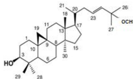
ترکیب ۳: سیکلوآرتان-۲۳-ان-۲۵-متواکسی-۳- \beta - \text{OH}
