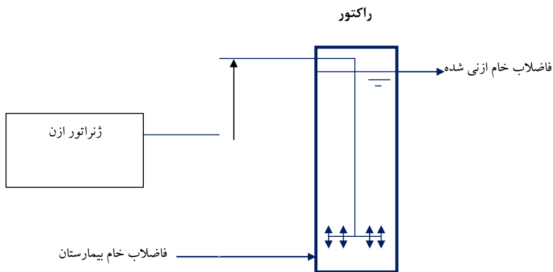
شکل ۱- راکتور مورد استفاده برای ازن زنی فاضلاب خام بیمارستان
