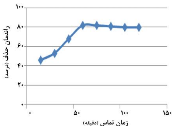
نمودار ۷ - تأثیر زمان تماس بر میزان جذب رنگ اورانژ ۷ با جاذب NH_2-MCM-41 در نمونه سینتتیک ( pH=4 و مقدار جاذب ۱۰ گرم در لیتر)
