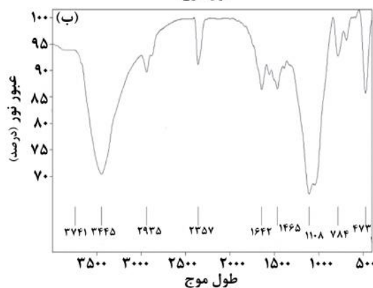
شکل ۲ - FTIR (الف) MCM-41 و (ب) نانوحفره NH 2 -MCM-41
