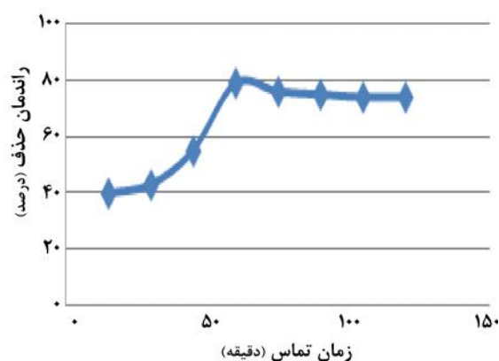
نمودار ۸ - تأثیر زمان تماس بر میزان جذب رنگ اورانژ ۷ با جاذب NH_2-MCM-41 در نمونه واقعی ( pH=4 و مقدار جاذب ۱۰ گرم در لیتر)
