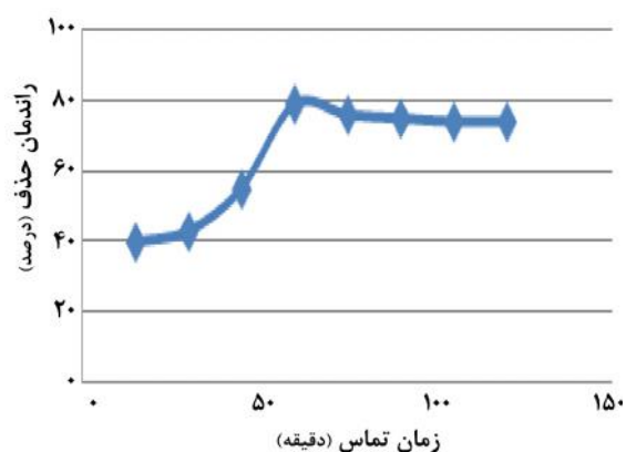
نمودار ۸ - تأثیر زمان تماس بر میزان جذب رنگ اسید اورانژ ۷ با جاذب NH_2 -MCM-41 در نمونه واقعی ( pH=4 ) و مقدار جاذب ۱۰ گرم در لیتر
