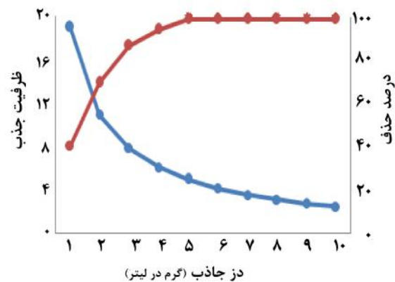
نمودار ۵- تأثیر دوز جاذب بر روی کارایی حذف (غلظت پنی‌سیلین G=25 میلی‌گرم در لیتر، زمان تماس ۷۵ دقیقه، pH=3 )
