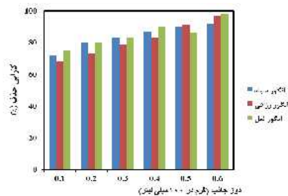
شکل ۲- تأثیر دوز جاذب بر کارایی حذف کروم شش ظرفیتی با استفاده از هسته‌های سه نوع انگور از محلول‌های آبی
