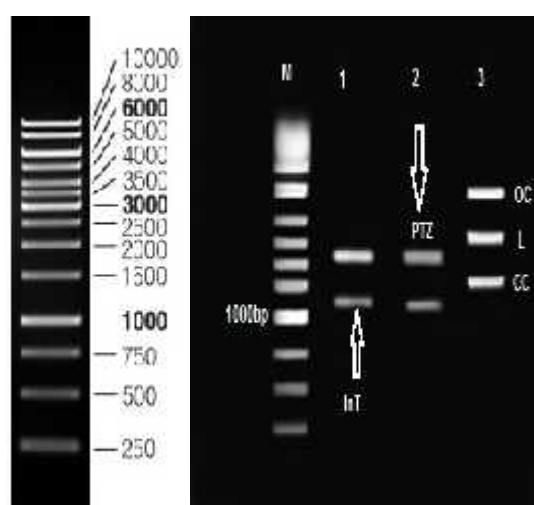
شکل ۲- نتیجه هضم آنزیمی روی پلاسمید pTZ-InT
