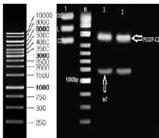
شکل ۳- نتیجه هضم آنزیمی روی پلاسمید نوترکیب pEGFP-C2-InT
