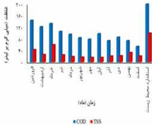
نمودار ۴- غلظت COD و TSS پساب خروجی حوض کلرزنی
