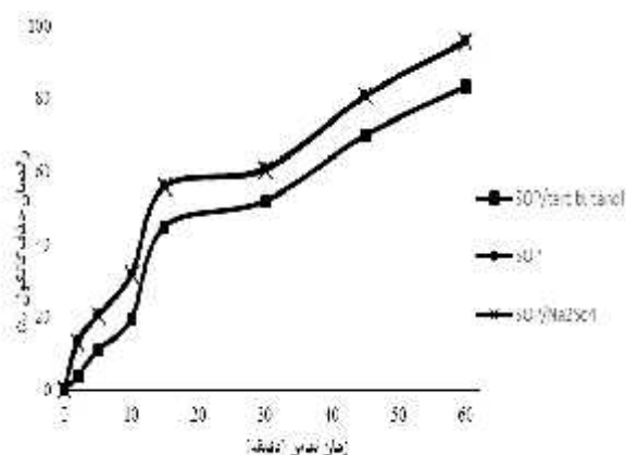
نمودار ۴- تأثیر به‌دام انداز رادیکال بر راندمان حذف کاتکول در فرآیند ازن‌زنی (غلظت کاتکول ۱۰۰۰ میلی گرم در لیتر، pH=۱۰، دوز ازن ۰/۳۸ گرم بر ساعت)
