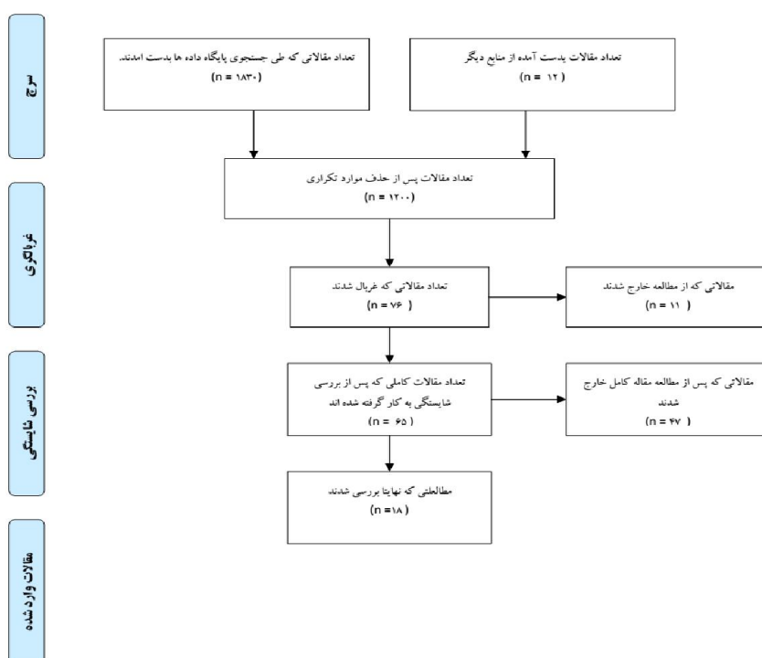
شکل ۱- فلوچارت PRISMA
