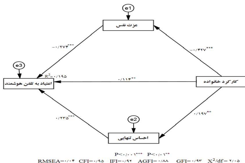
شکل ۲- مدل نهایی اعتیاد به تلفن هوشمند بر اساس کارکرد خانواده، عزت نفس و احساس تنهایی به همراه ضرایب استاندارد در دانش‌آموزان پسر شهر تهران در سال تحصیلی ۱۴۰۰-۱۳۹۹
