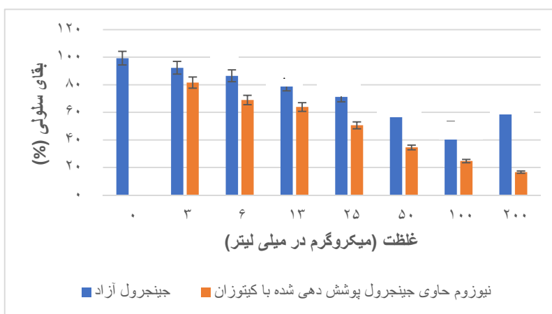
نمودار ۵- ارزیابی درصد بقاء سلولی رده سلولی سرطان پستان پس از تیمار با نیوزوم‌های حاوی جینجرویل و جینجرویل آزاد. نمودار به صورت انحراف معیار \pm میانگین رسم شده است. اختلاف معناداری در مقایسه با گروه کنترل (غلظت ۰) در نظر گرفته شده است.
