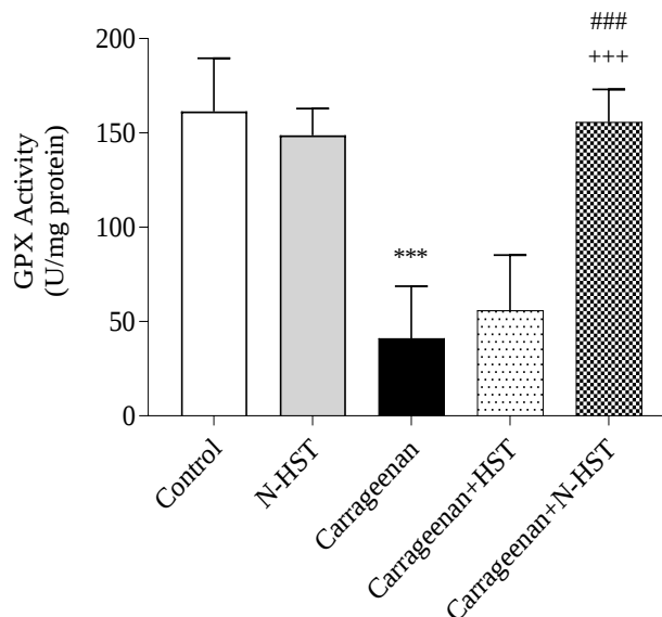
نمودار ۴- بررسی فعالیت آنزیم گلوکوتاتیون پراکسیداز در بافت پنجه پای موش
