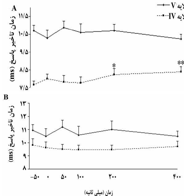
نمودار ۳- اثر تحریک الکتریکی هسته رافه خلفی در زمان‌های مختلف (صفر تا ۴۰۰ میلی ثانیه) قبل از جا به جایی مکانیکی سبیل اصلی (A) و کناری (B) بر زمان تأخیر پاسخ نورون‌های لایه IV و V. فاصله زمانی (۰-۵۰- تا صفر) میلی ثانیه اثر جا به جایی مکانیکی سبیل کناری به تنهایی و بدون تحریک الکتریکی هسته رافه خلفی می‌باشد. اعداد نشان دهنده میانگین \pm خطای معیار می‌باشند (*: p < 0.05 و **: p < 0.01 ).
