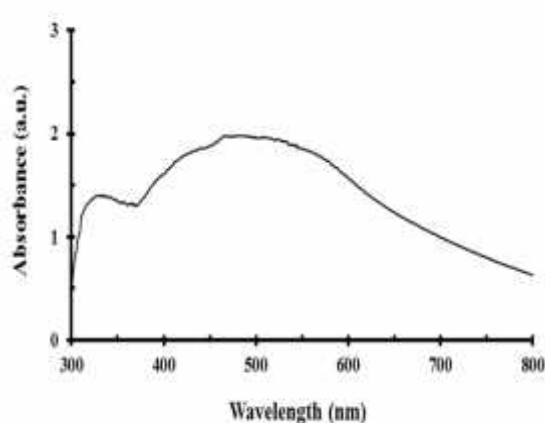
شکل ۲- طیف UV-visible نانوذرات سلنیوم بیوژنیک
