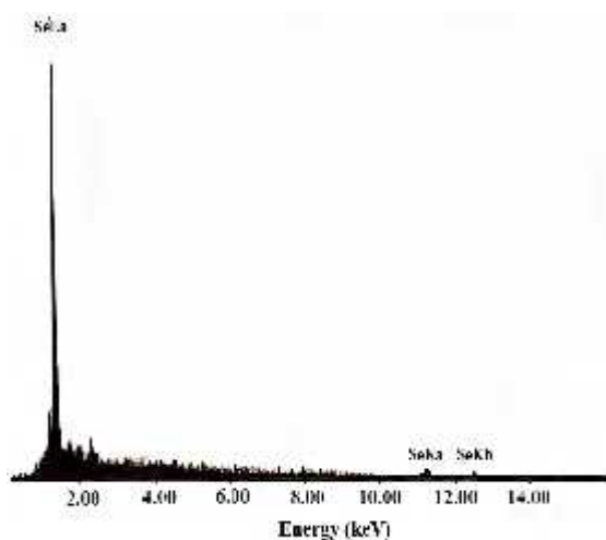
شکل ۵- طیف EDX نانوذرات سلیوم بیوژنیک
