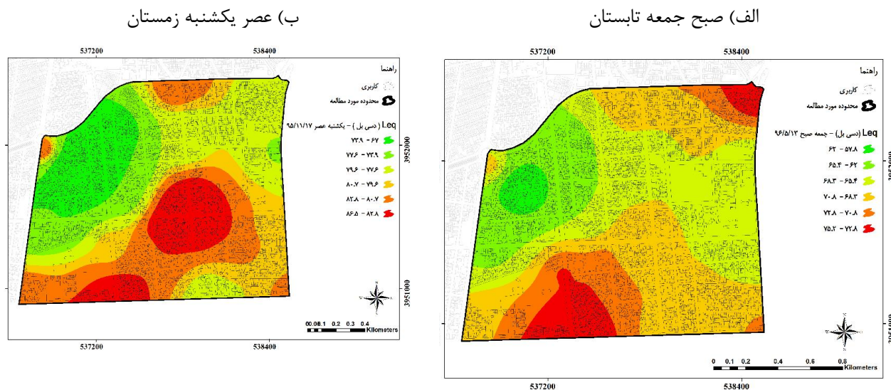
شکل ۲- توزیع فضایی شاخص L_{eq} در (الف) خلوت‌ترین و (ب) شلوغ‌ترین روزها و ساعات هفته در ناحیه یک- منطقه شش تهران (۹۶-۱۳۹۵)
