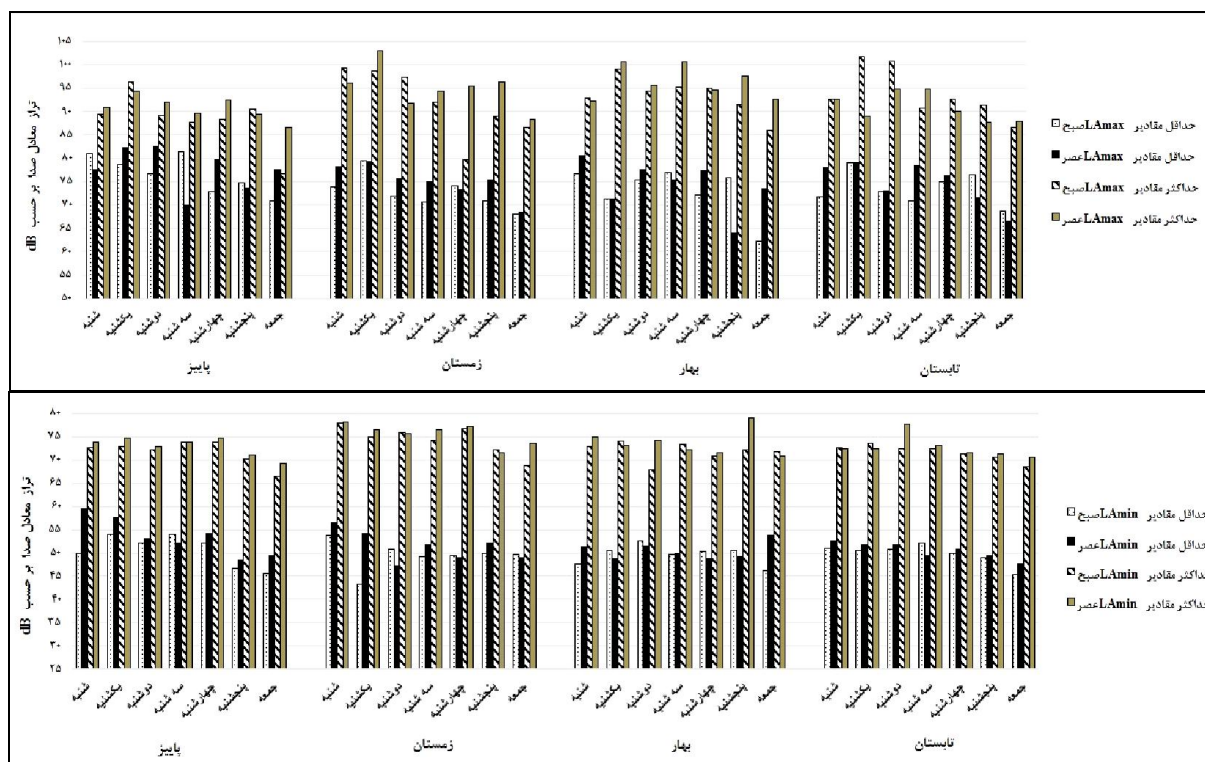
نمودار ۱- حداقل و حداکثر مقادیر L_{max} و L_{min} بر حسب دسی بل در ساعات اوج ترافیک صبح و عصر در ناحیه یک- منطقه شش تهران (۹۶-۱۳۹۵)
