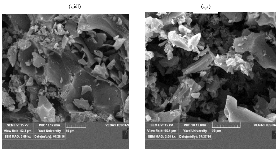
شکل ۲- تصاویر SEM کربن فعال گرانولی تجاری قبل از استفاده (الف) و بعد از جذب سطحی در زمان تماس بهینه ۱۵ دقیقه (ب)
