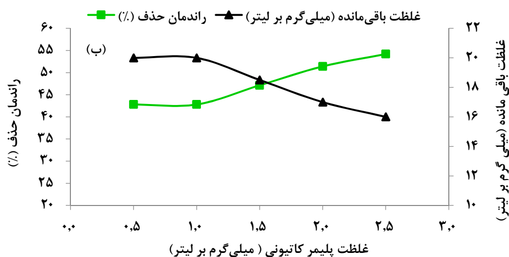
نمودار ۳- تأثیر غلظت های مختلف پلیمر آنیونی (الف) و پلیمر کاتیونی (ب) در حذف بور از فاضلاب ( pH=8 غلظت پلی آلومینیوم کلراید = 400 میلی گرم بر لیتر)
