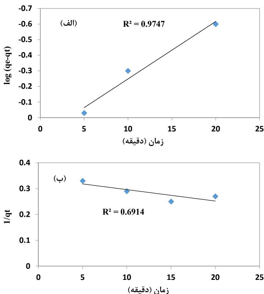
نمودار ۷- مدل‌های سینتیک شبه درجه اول (الف) و شبه درجه دوم (ب) برای جذب بور
