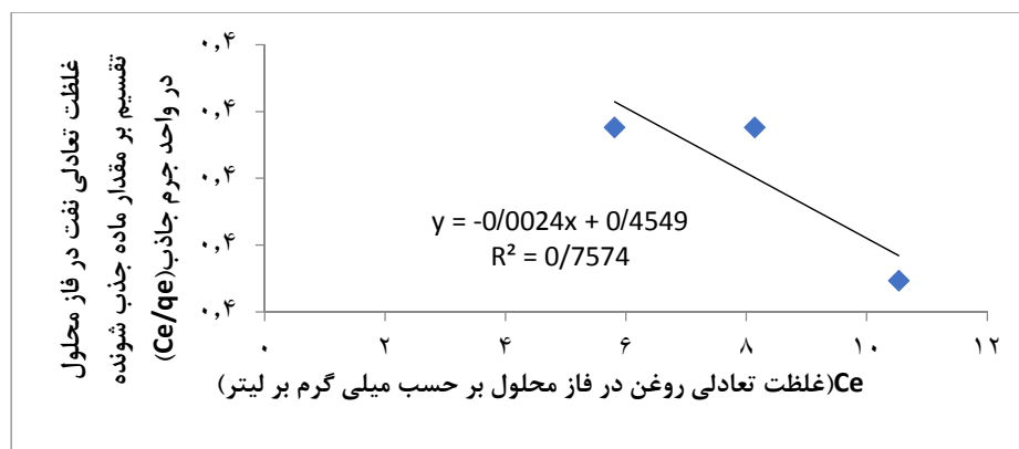
نمودار ۲- هم‌دم‌های جذبی Langmuir جذب جذب نفت به وسیله جاذب نانو ذره اکسید روی سنتز شده
