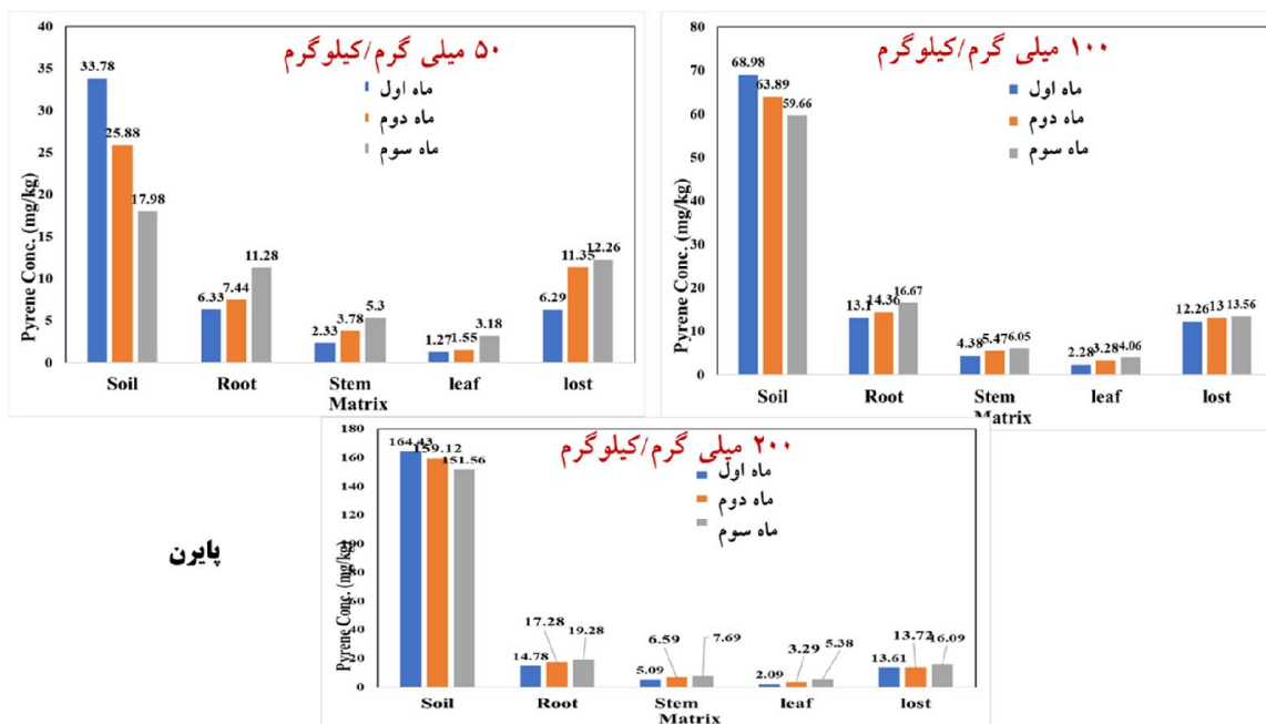
شکل ۲- کارآبی فرآیند گیاه پالایی با استفاده از درخت کهور در حذف پیرن از خاک رس آلوده حاوی سورفکتانت و کود حیوانی
