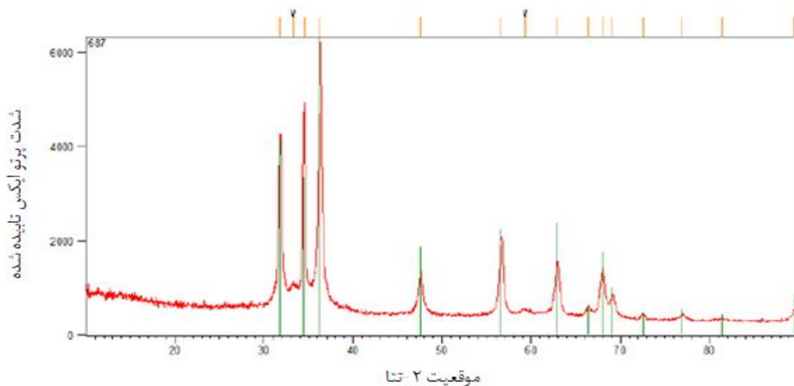
شکل ۶- آنالیز XRD نانوذرات اکسید روی سنتز شده. نتایج XRD نشان دهنده سنتز نانوذرات اکسید روی می‌باشد. الگوی طیف به دست آمده از ویرایش اشعه ایکس در زاویه \theta دارای پیک‌های ۰۴۶/۵۶، ۰۳۶/۲۹، ۰۳۴/۴۵، ۰۳۳/۲۸، ۳۳/۸ بود که با الگو پراش اشعه ایکس ZnO مطابقت دارد.
