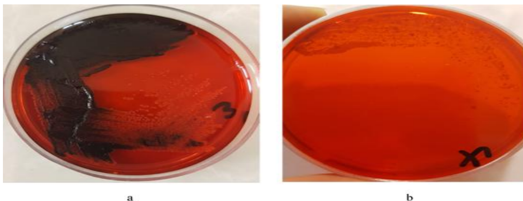
شکل ۸- تست تشکیل بیوفیلم در محیط کشت کنگورد آگار. سویه‌های تشکیل دهنده بیوفیلم در محیط کشت کنگورد آگار کلنی مشکی رنگ (a) و سویه‌های بیوفیلم منفی کلنی‌های سفید رنگ تشکیل می‌دهند (b).
