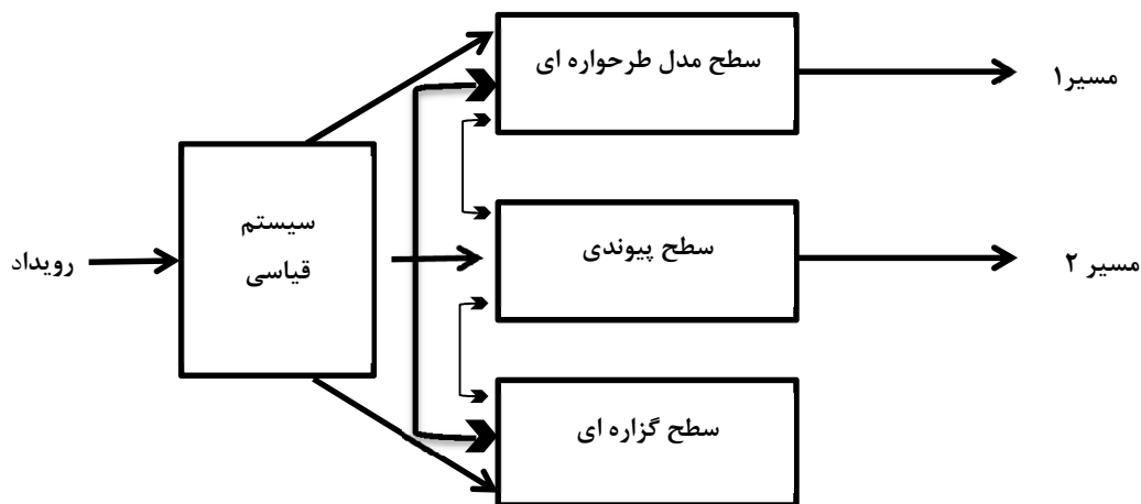
شکل ۱- مدل اسپارس
