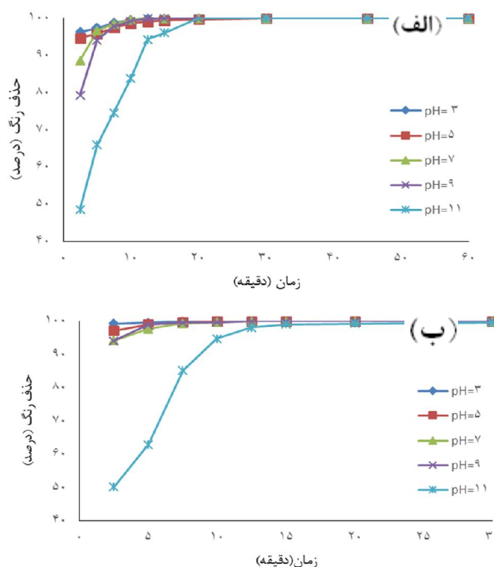
نمودار ۱-الف: تأثیر pH محیط بر الف: کارایی فرآیند UV/SrO_8 و ب: کارایی فرآیند UV/H_2O_2 در حذف رنگ اورانین (غلظت اولیه رنگ ۵۰ میلی‌گرم در لیتر؛ دوز پرسولفات ۱ میلی‌مول بر لیتر؛ دوز پراکسید هیدروژن ۲۰ میلی‌مول بر لیتر)
