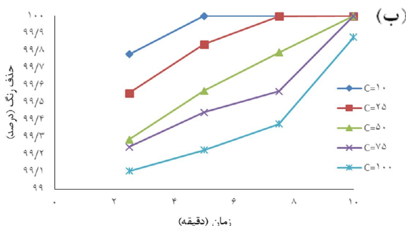
نمودار ۳- الف: تأثیر غلظت اولیه رنگ اورانین بر کارایی فرایند UV/S 2 O 8 و ب: کارایی فرایند UV/H 2 O 2 (pH=3) پرسولفات ۲ میلی مول بر لیتر؛ پراکسید هیدروژن ۲۰ میلی مول بر لیتر)
