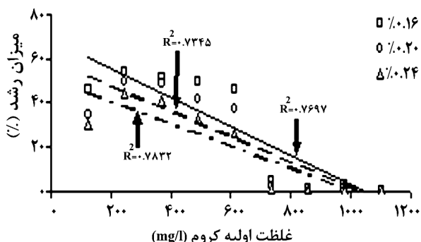
نمودار ۷: میزان حذف کروم با توجه به غلظت‌های اولیه کروم در پساب و مقادیر مختلف تلقیح قارچ آسپرژیلوس نیجر
