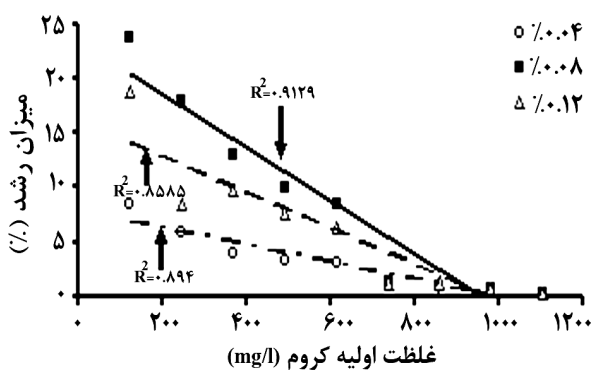
نمودار ۴: نسبت وزنی توده رشد یافته به غلظت کروم در غلظت‌های مختلف کروم در پساب و مقادیر مختلف تلقیح
