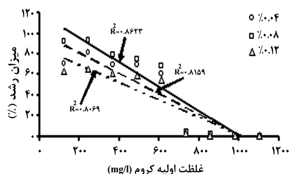
نمودار ۶: میزان حذف کروم با توجه به غلظت‌های اولیه کروم در پساب و مقادیر مختلف تلقیح قارچ آسپرژیلوس نیجر
