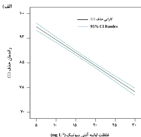
شکل ۴-الف) تأثیر غلظت اولیه آنتی‌بیوتیک بر راندمان حذف تتراسایکلین (pH برابر با ۷/۰، مقدار جاذب ۳ گرم در لیتر و زمان واکنش ۳۸ دقیقه)، ب) تأثیر همزمان غلظت اولیه آنتی‌بیوتیک و pH محلول بر راندمان حذف تتراسایکلین (مقدار جاذب برابر با ۳ گرم در لیتر و زمان واکنش ۳۸ دقیقه).
