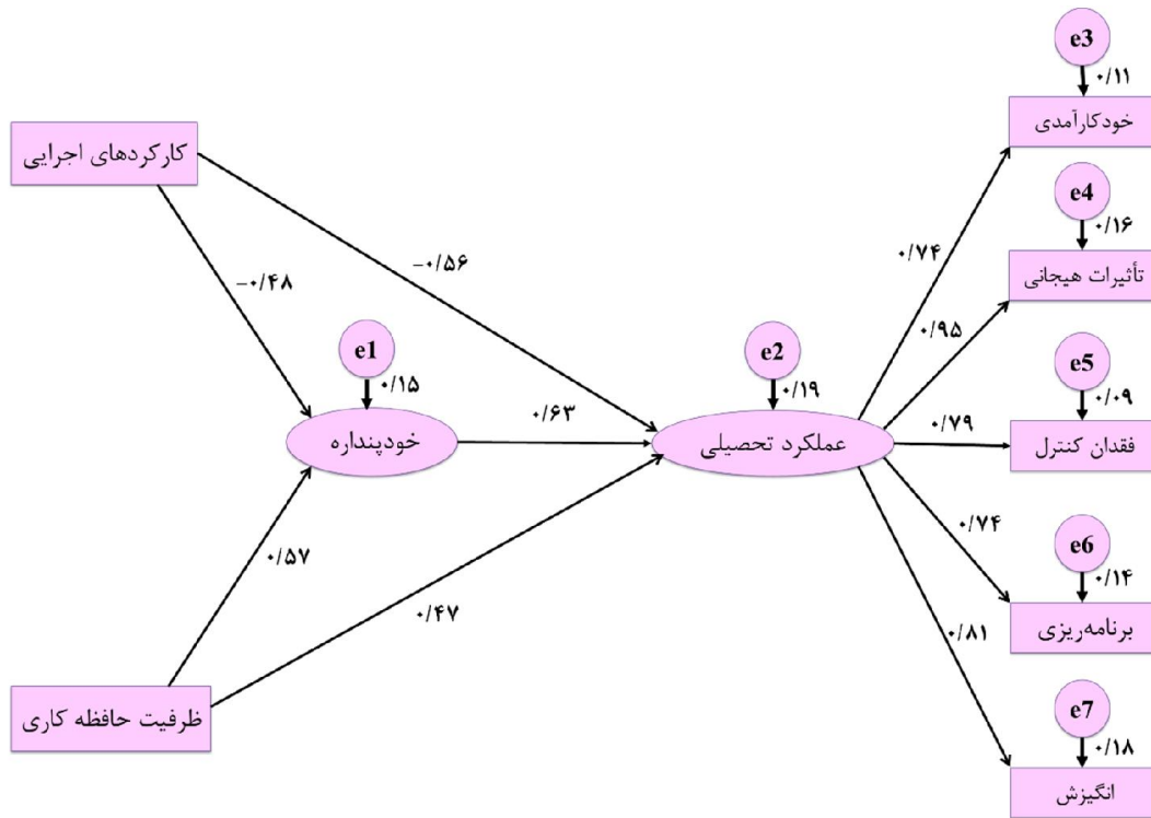
شکل ۲- تحلیل مسیر نقش میانجی خودپنداره در رابطه تقابص کارکردهای اجرایی و ظرفیت حافظه کاری با عملکرد تحصیلی دانش‌آموزان دوره اول دبیرستان سمیرم ( P < 0.05 به عنوان سطح معناداری).
