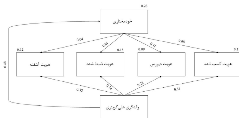
شکل ۱- مدل دیداری ضرایب به دست آمده برای ارتباط بین رابطه والدگری هلی کوپتری و هویت یابی در نوجوانان با نقش واسطه گری خودمختاری در دانش آموزان متوسطه استان تهران در سال ۱۴۰۲ (n=۲۰۷)
