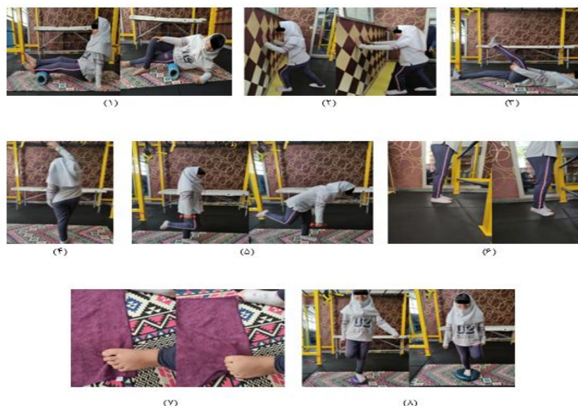
شکل ۷- تمرینات اصلاحی تحقیق حاضر شامل: رها سازی عضلات دوقلو/نعلی و کشنده پهن نیام با استفاده از فوم رول توسط خود فرد (تمرین ۱)، کشش عضله دوقلو/ نعلی (تمرین ۲)، کشش عضله دوسرانی (تمرین ۳)، کشش عضله کشنده پهن نیام (تمرین ۴)، حرکت ددلیفت تک پا (جهت تقویت عضله ساقی قدامی) (تمرین ۵)، بالابردن ساق پا (حرکت روی پنجه جهت تقویت عضلات خلفی ساق پا) (تمرین ۶)، جمع کردن حوله با پا (جهت تقویت عضلات درون کف پای) (تمرین ۷) و دست یابی به تعادل روی یک پا در چند سطح (تمرین ۸)
