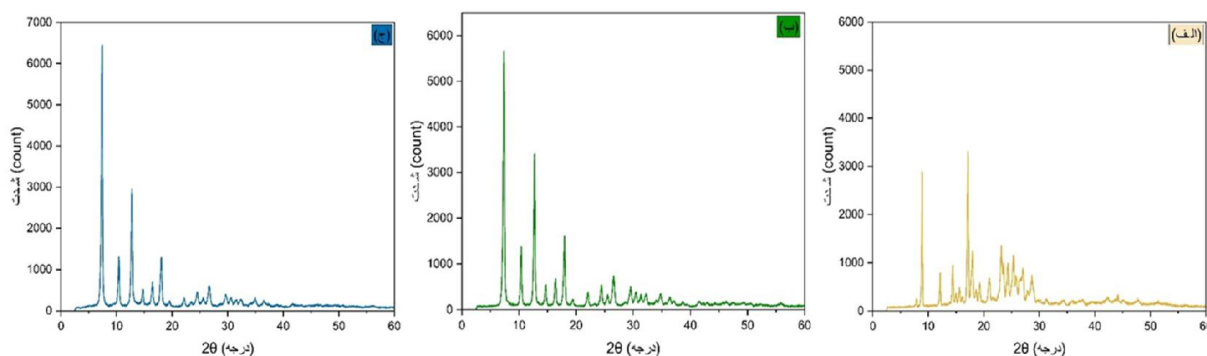
شکل ۴- الگوی پراش اشعه ایکس برای (الف) کورکومین (ب) نانوذره ZIF-8 (ج) نانوذره CUR@ZIF-8
