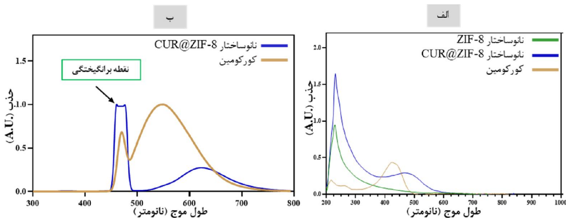
شکل ۵- نمودارهای طیف سنجی (الف) مرئی-ماوراء بنفش (ب) فوتولومینسانس
