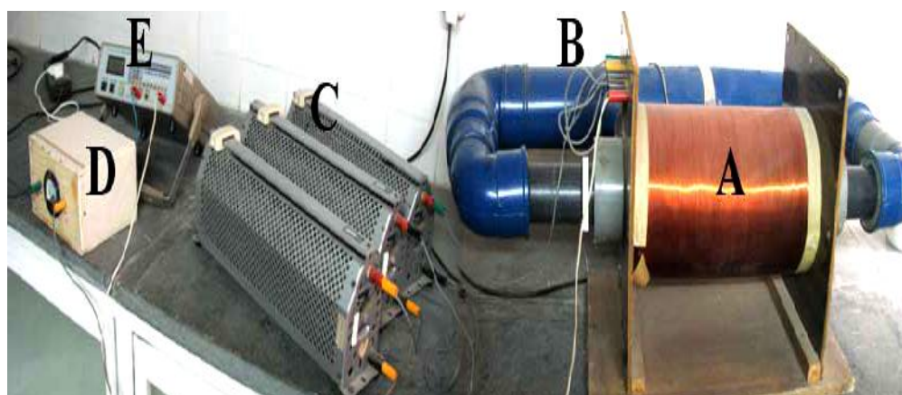
شکل ۱- سیستم مولد میدان الکترومغناطیس و اتکوباسیون. A سیم پیچ مولد میدان الکترومغناطیس، B محفظه اتکوباسیون، C رئوستا، D خازن، E ولت‌سنج.
