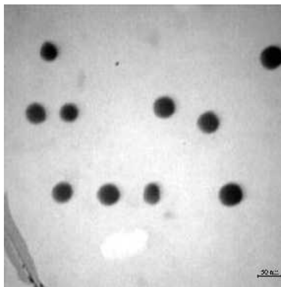
شکل ۳- تصویر میکروسکوپ الکترونی TEM نانوذرات سلینیوم بیوژنیک
