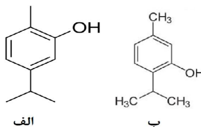
شکل ۱- فرمول ساختاری ترکیبات اصلی گیاه آویشن. الف) کارواکرول، ب) تیمول
