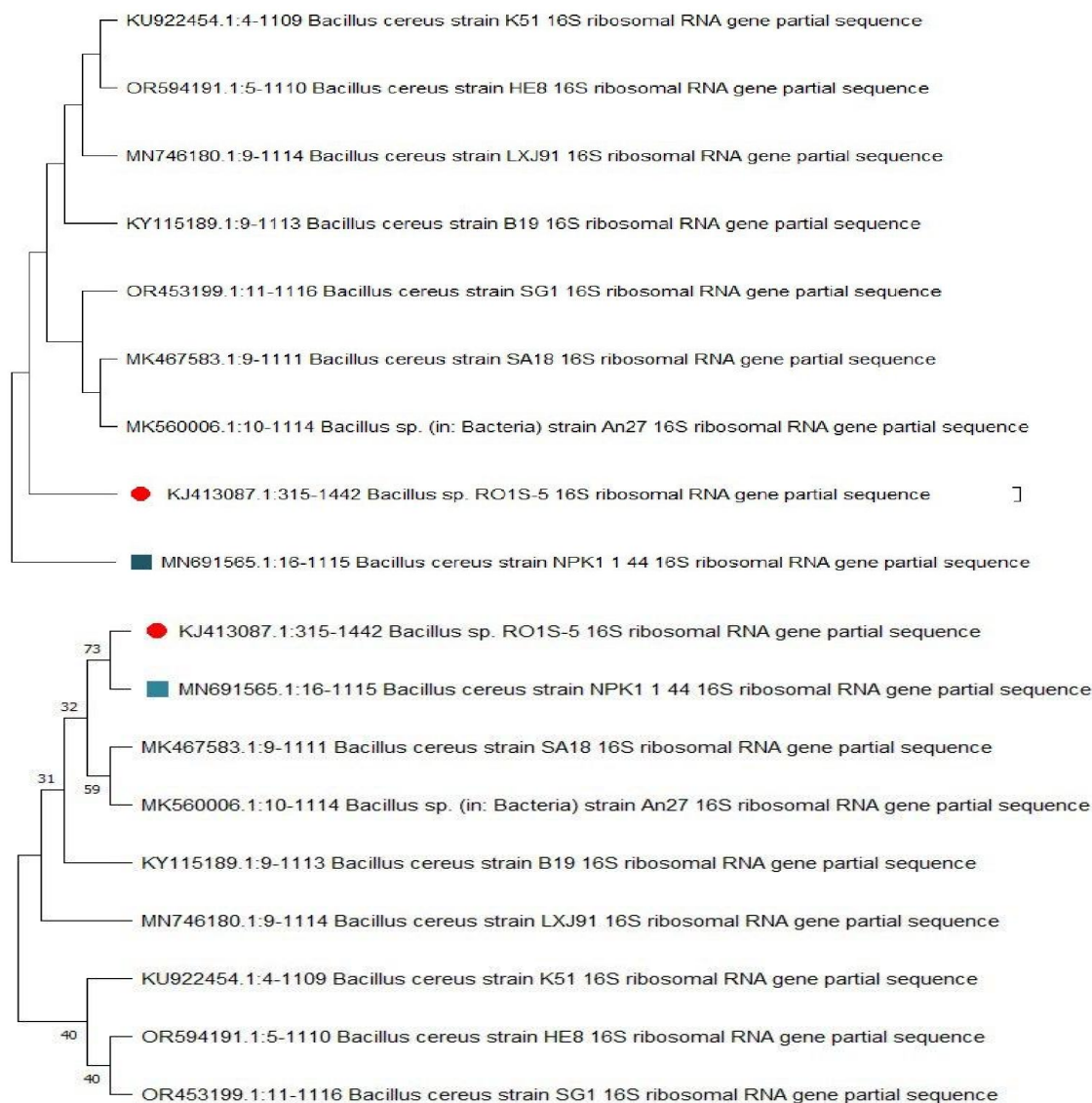
شکل ۱- درخت فیلوژنتیکی
